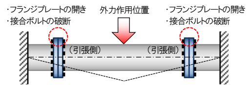
a) フランジ継手直撃型(下流視)
