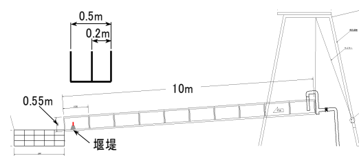
図-4 実験水路の縦断面図
