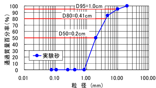
図-5 実験砂の粒度分布
