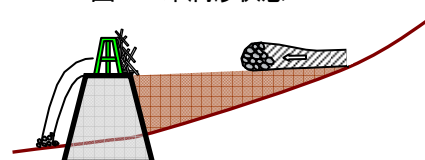
図-2 満砂状態
