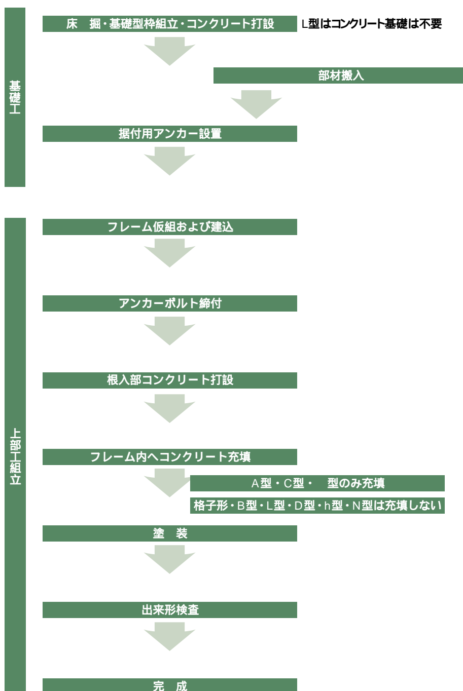
図2 鋼製透過型砂防えん堤の一般的な施工手順
